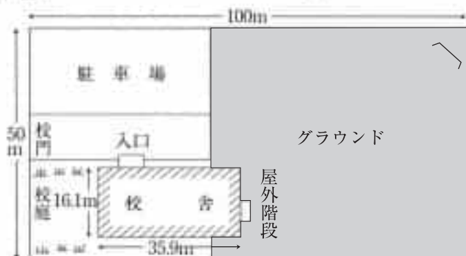
(2) 校舎配置図
